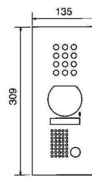
Encastrement (115 x 282 x 45 mm) Platine de rue encastrée avec clavier à code
