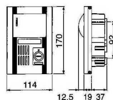
Boîtier d'encastrement (155 x 95 x 65 mm)
